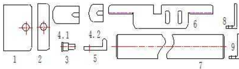
图 10 压力仪测量附件示意图(附件 5 已去掉)
