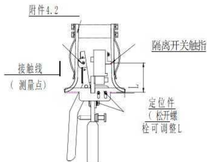
图 8 转入式触头隔离开关压力测量示意图
