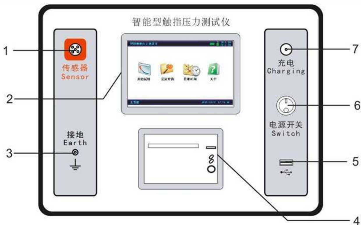
图 1 面板布置图
