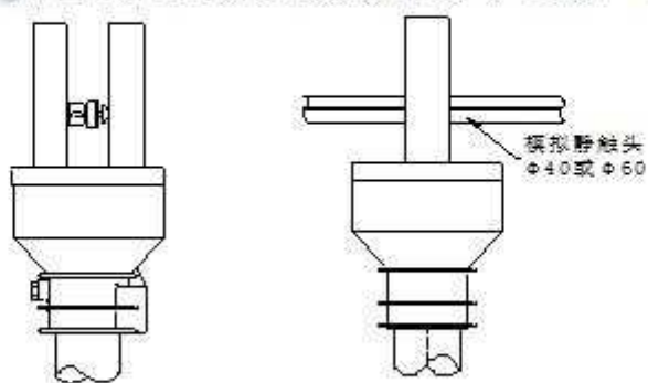
图13 折臂式隔离开关用模拟触头测量示意图
