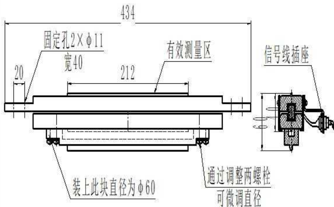
图12 折臂式隔离开关模拟触头（ \Phi 40 、 \Phi 50 、 \Phi 60 ）
